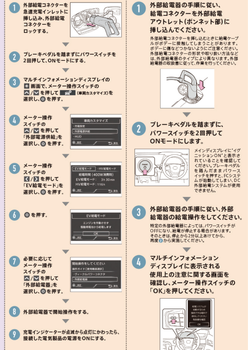
外部給電アウトレット (ボンネット下コンパートメント内)
